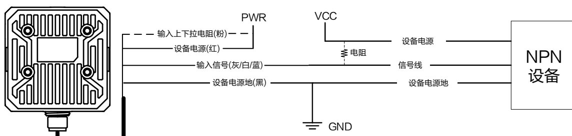
图5-10 输入信号接 NPN 设备
