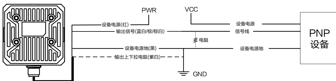
图5-15 输出信号接 PNP 设备
