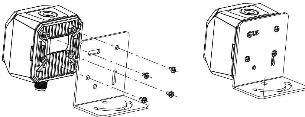
图3-2 安装方式二
