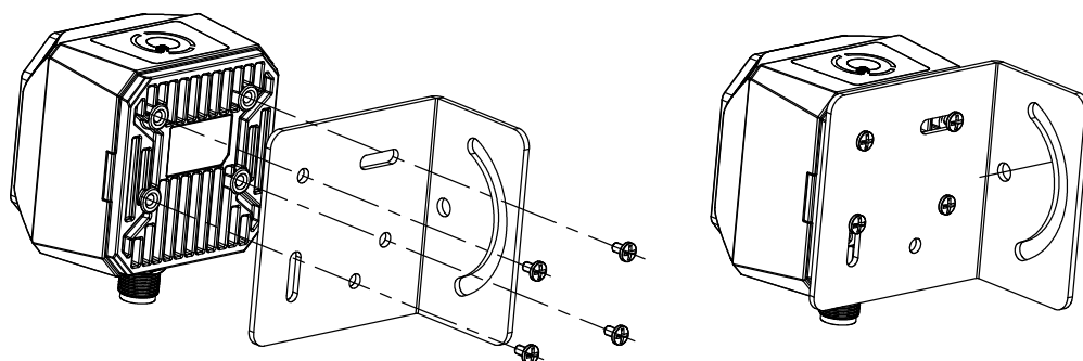
图3-1 安装方式一
